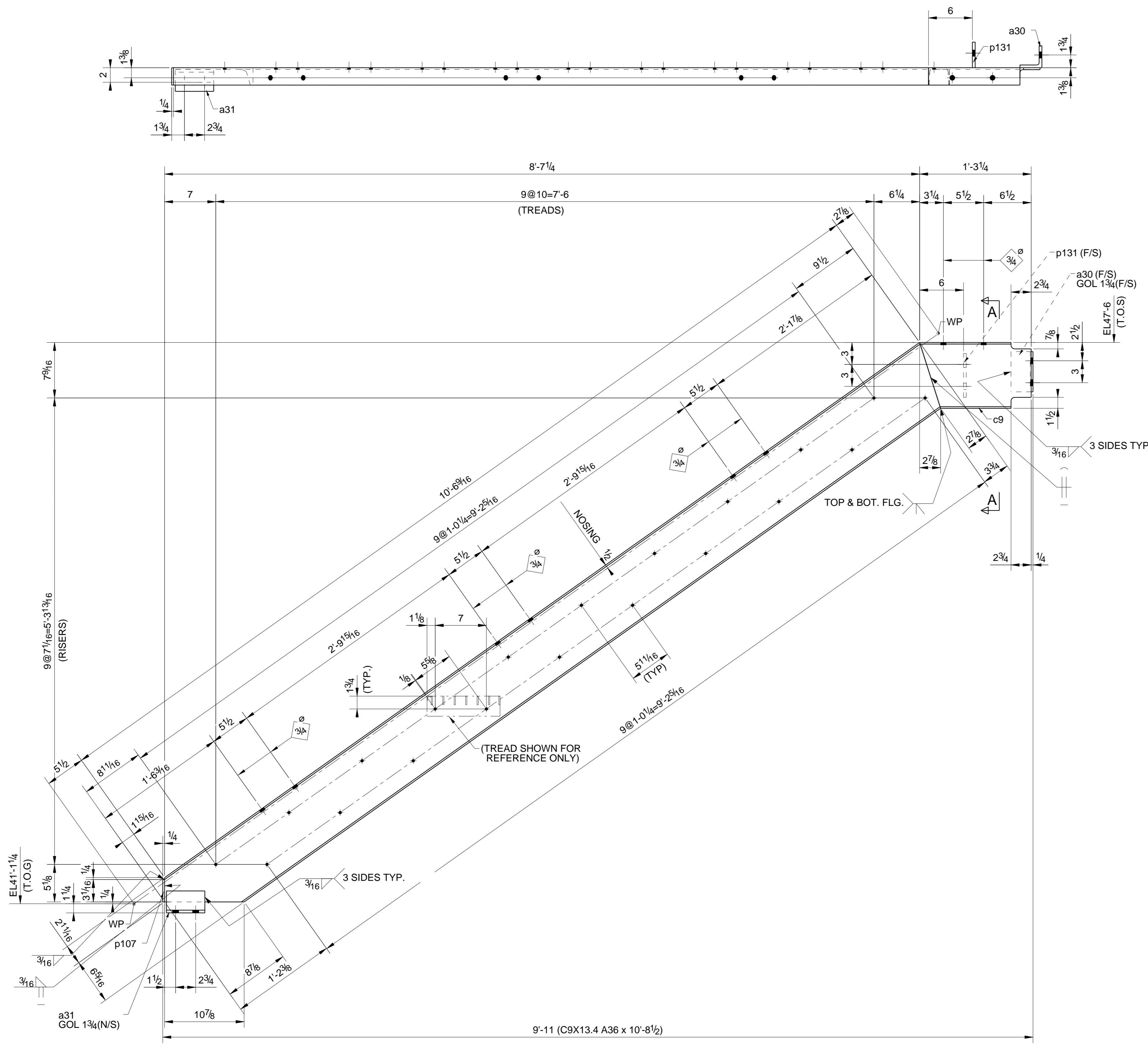
2 - STRINGERS - 41S1 1326
