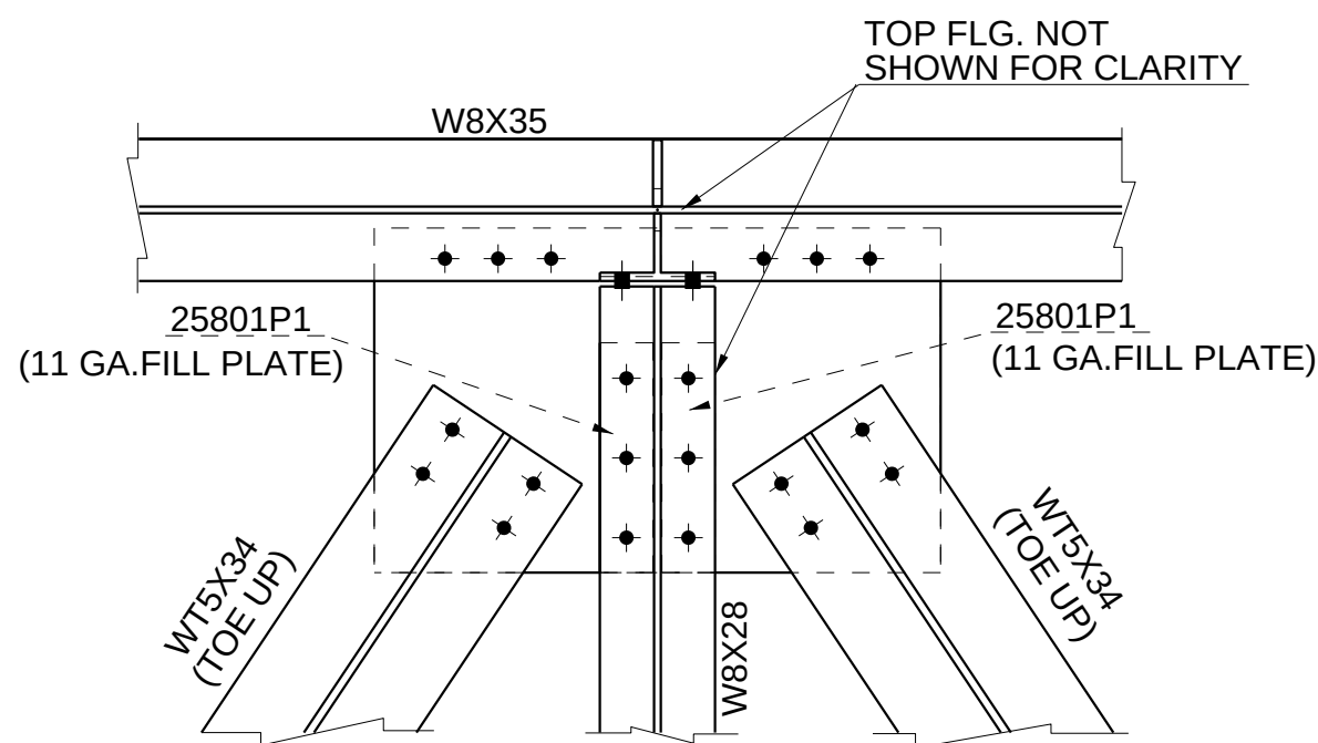
DETAIL G E25005
