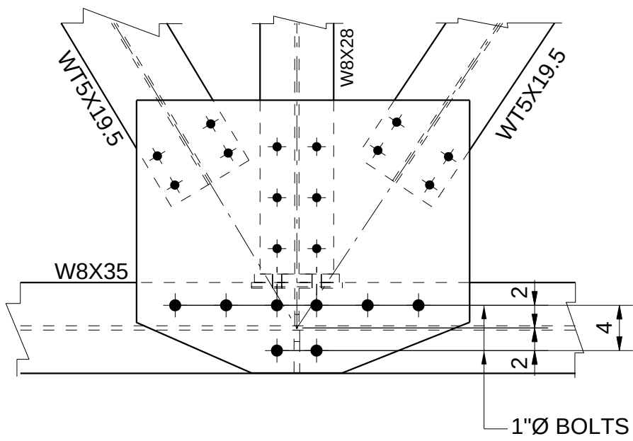
DETAIL F E25005
