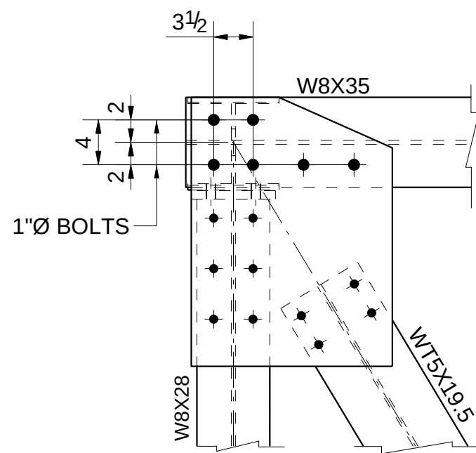
DETAIL D E25005
