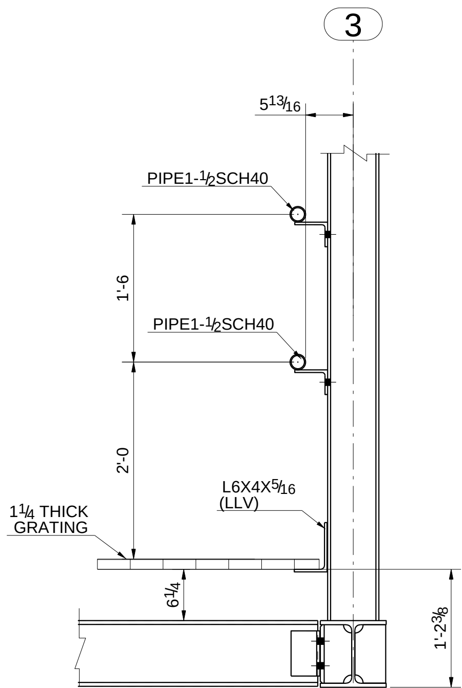
DETAIL C E25007
